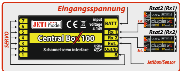
Fig. 11: Blockschaltbild der Central Box 100 Verbindungen - EX Bus Variante
