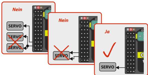
Fig. 8: Korrekter Anschluss der Servos an die Central Box
