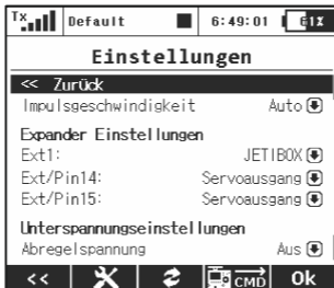
Fig. 15: Geräteübersicht-HauptEinstellungen
