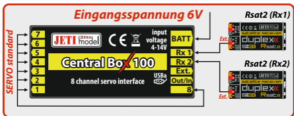
Fig. 5: Beispiel für den Einsatz der Central Box 100 mit Standardservos (max. Spannung für die Servos 6V)
