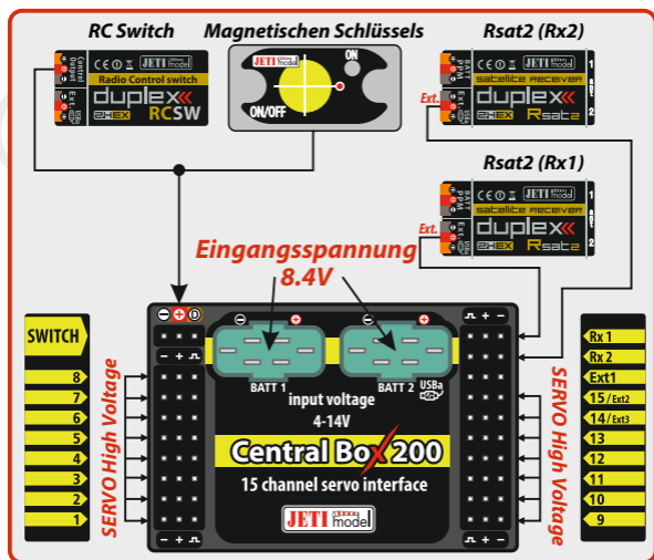
Fig. 6: Beispiel für den Einsatz der Central Box 200 mit HV-Servos (HIGH Voltage Servos)
