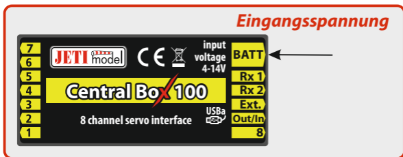
Fig. 2: Central Box 100 Beschreibung
